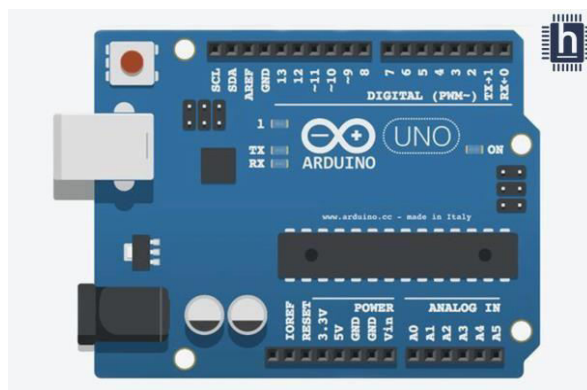
Fig. 1. Arduino UNO
