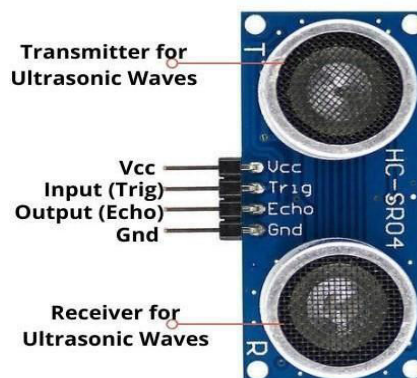
Fig. 3. HC-S304Ultrasonic Sensor
