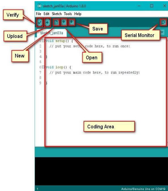
Fig. 2. Arduino Software (IDE)
